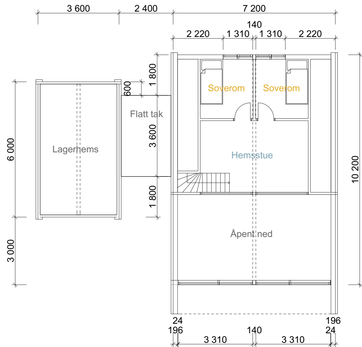
1:100 Hems
