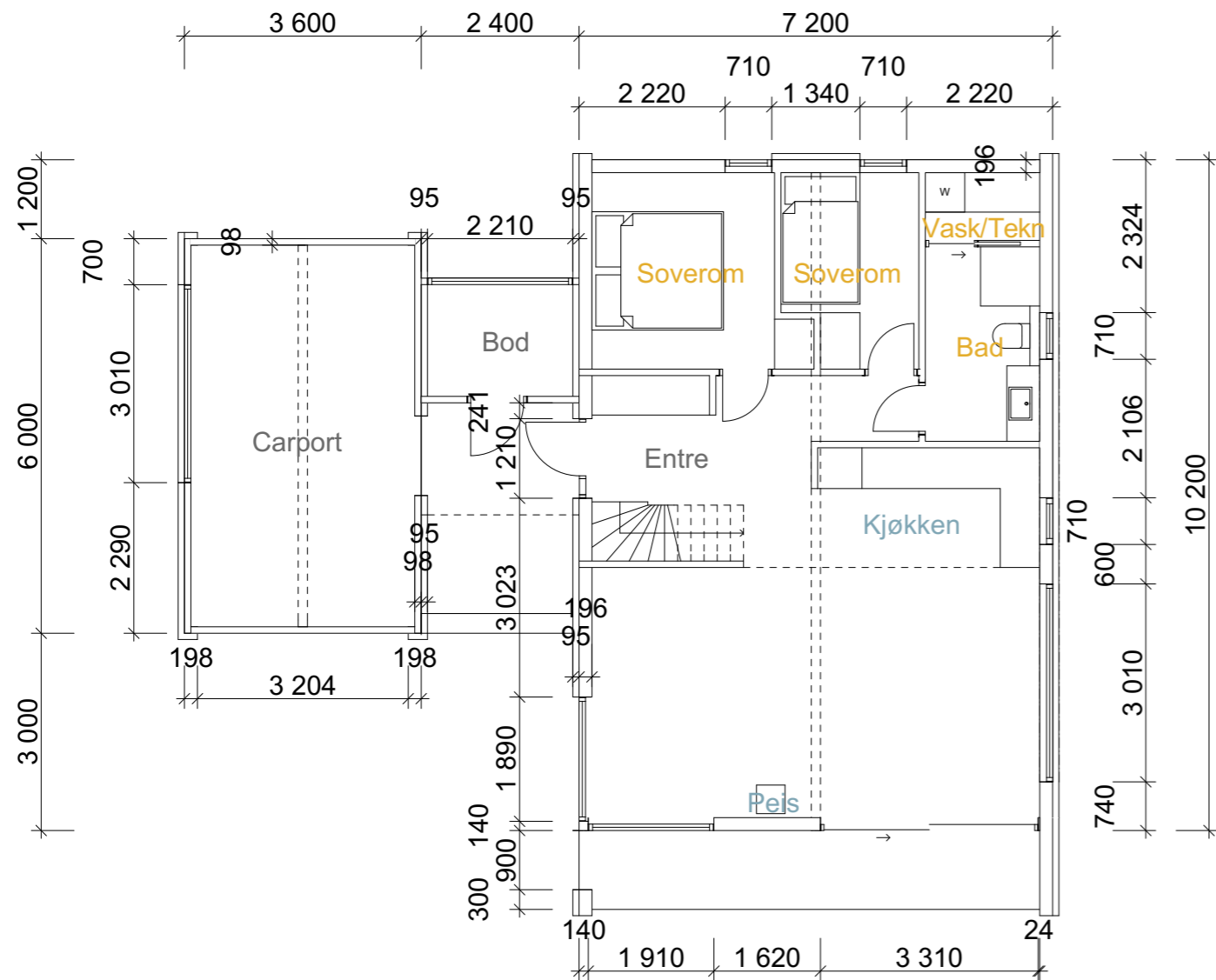
1:100 1. Etasje
